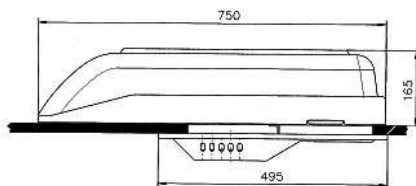
Seitenansicht mit Luftverteilerplatte
