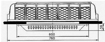
Frontansicht mit Luftverteilerplatte
